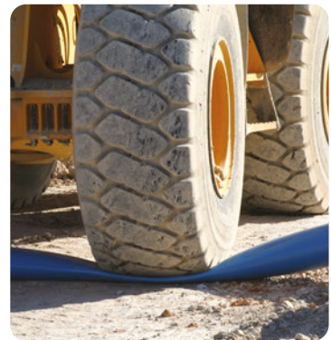
La tubería TOM® soporta las máximas deformaciones sin sufrir daños estructurales.
